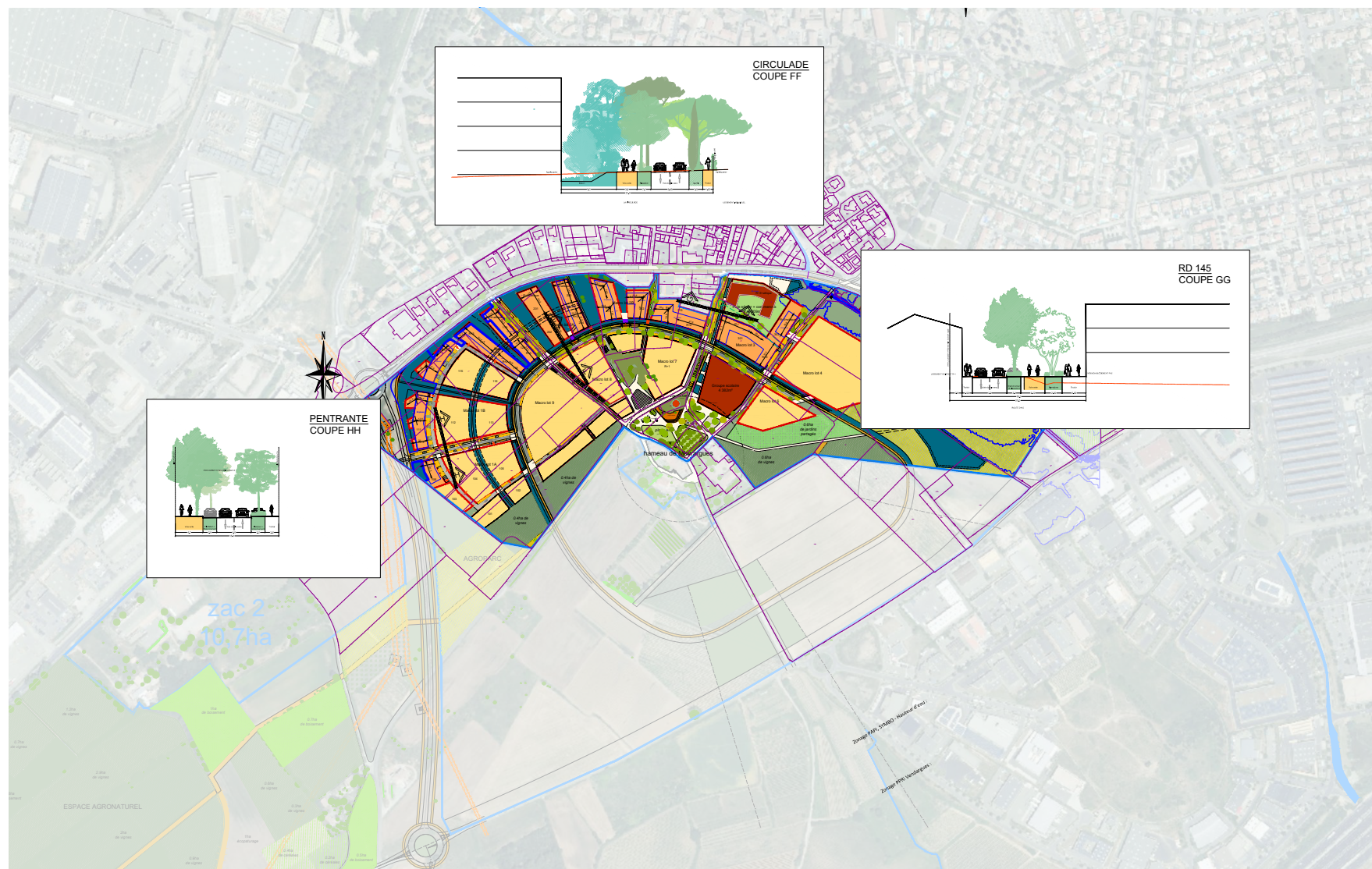
Équipements ZAC, voiries - GGL Aménagement, SERI, Agence APS, TOURRE-SANCHIS
