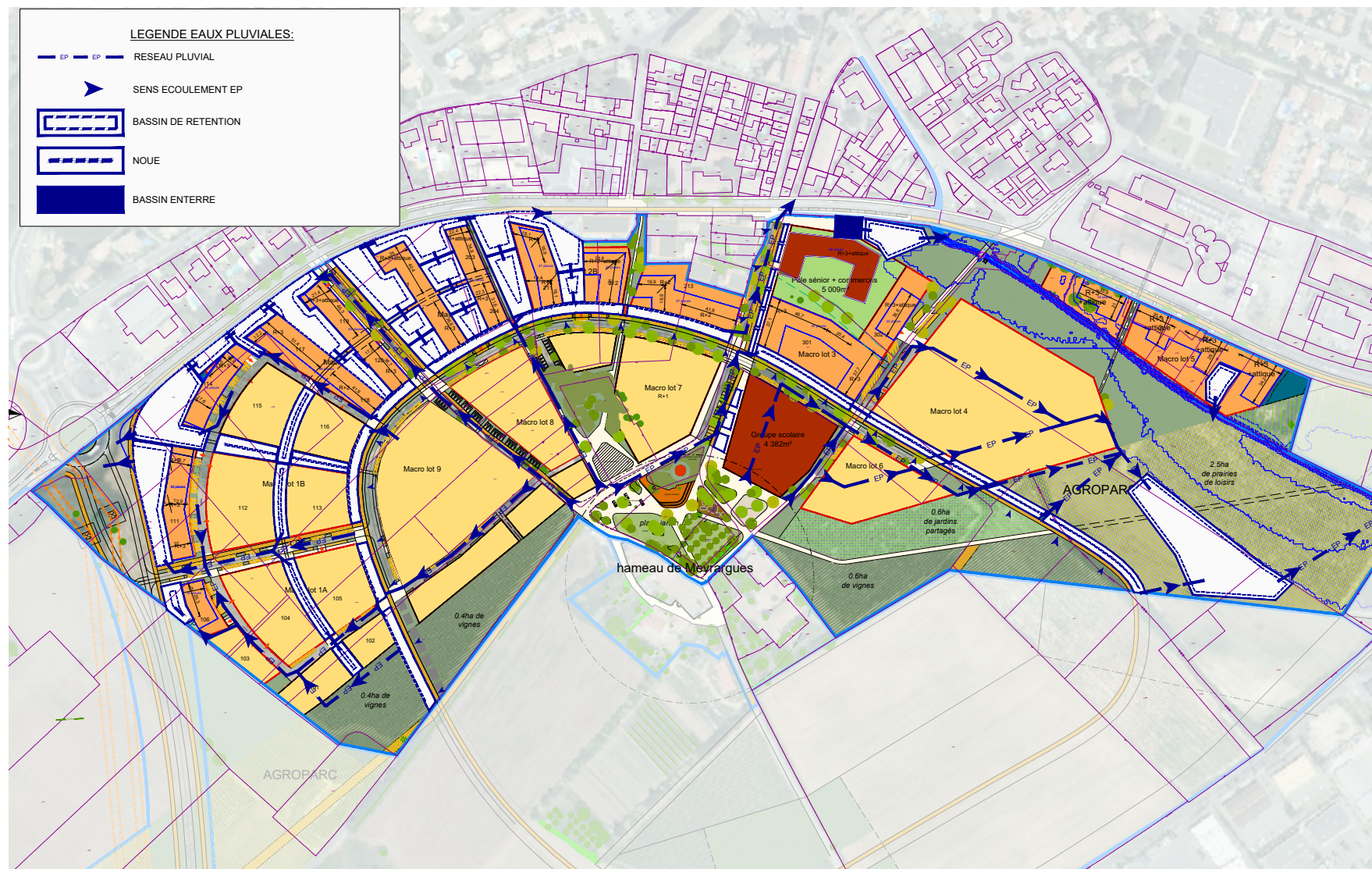
Schéma Directeur d'eaux pluviales (EP) - GGL Aménagement, SERI, Agence APS, TOURRE-SANCHIS
