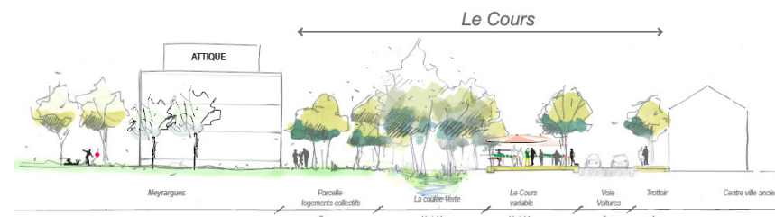
Coupe de principe sur le cours - Dossier de création de la ZAC Meyrargues
